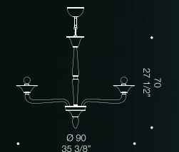
7086 K6 6xMAX 46W E14
