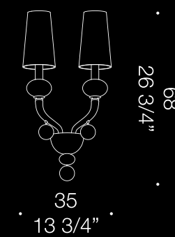
MADemoiselle A2 2xMAX 46W E14
