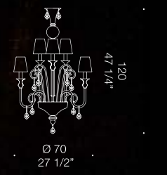
BUGIA K8 8xMAX 46W E14
