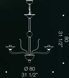
7077 K8 8xMAX 46W E14
