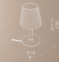
LUMÈ L 1xMAX 46W E14
