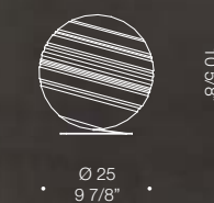
STRATOSFERA L25 1xMAX 77W E27 tubolar
