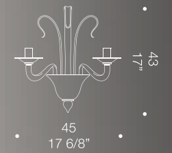
7088 A2 2xMAX 46W E14
