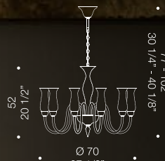
2612 K10 10xMAX 46W E14
